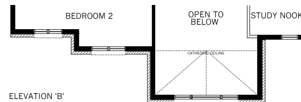
ELEVATION 'B'
